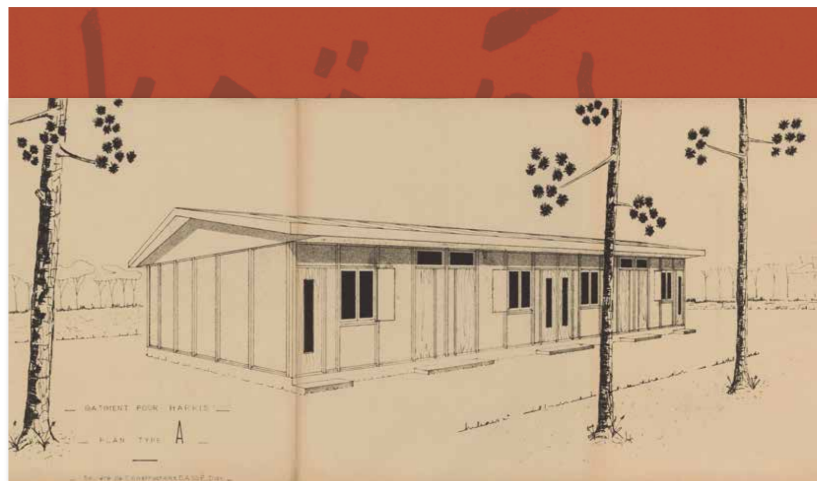
Vue cavalière d'un préfabriqué construit à Rosans pour servir de logement aux familles de harkis, 1964 (242 W 7006).
